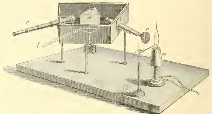
Nr. 5060. Des Kirchhoff- und Bunsen'sche Spektroskop.
