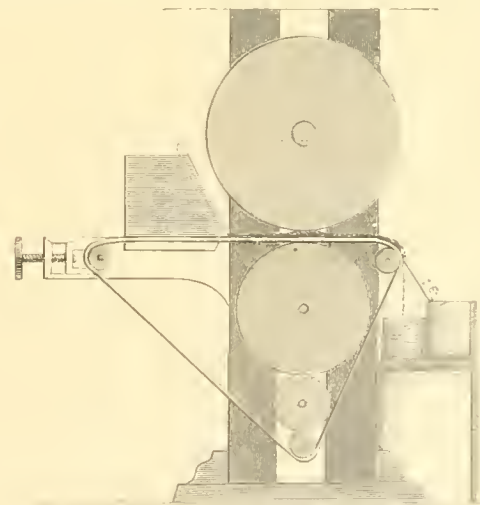
Nr. 4812. Preussische Pulverpresse.
