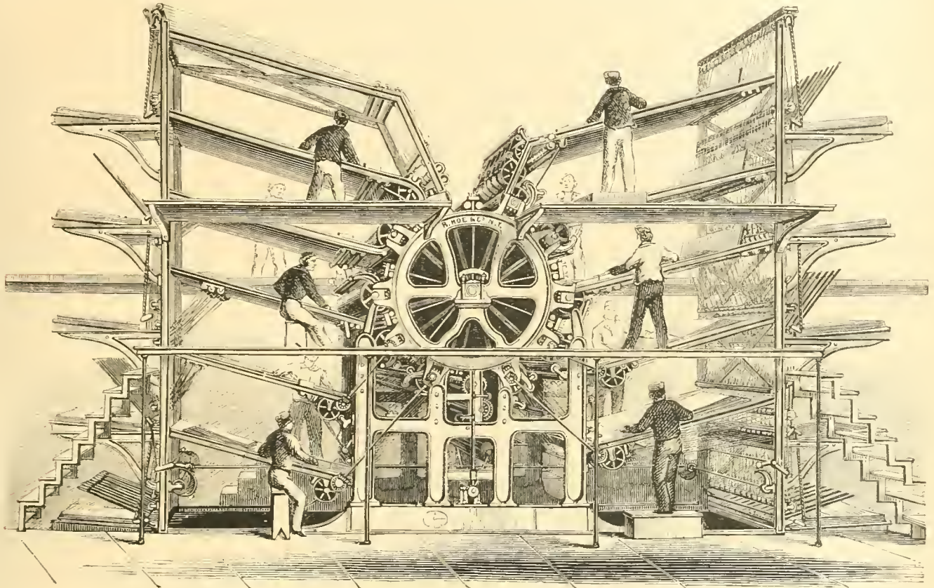
Nr. 4887. Hoe's Maschine mit einem Typen- und zehn Druckcylindern (Type revolving Machine).
