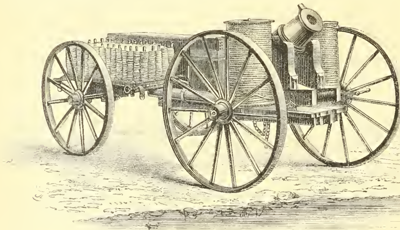
Nr. 4611. Bombenbatterie zur Rettung Schiffbrüchiger.
