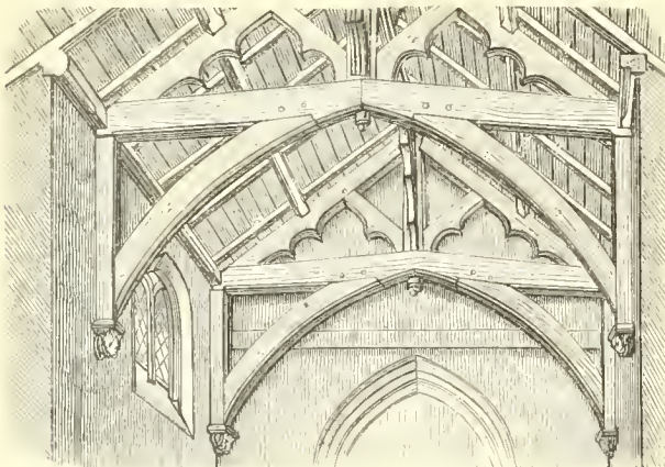
Nr. 5097. Dachstuhl mit Häng- und Sprengwerk aus Addeburg (14. Jahrh.).
