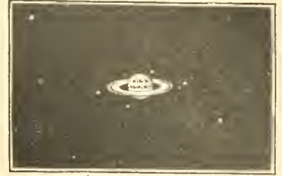
Nr. 4773. Saturn und seine Trabanten.
