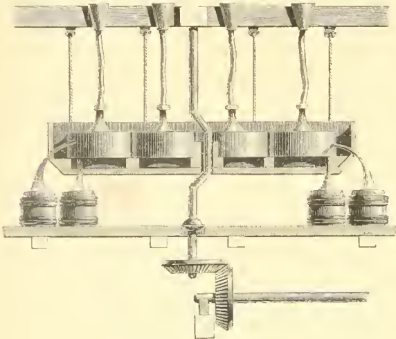
Nr. 1513. Körnmahlmaschine.
