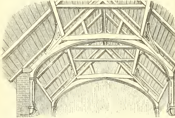
Nr. 5096. Dachstuhl mit Sprengwerk aus St. Mary in Leicester (13. Jahrh.).
