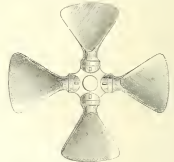
Nr. 4903. Viergängige Schraube des Rennie's Fischschwanzform.
