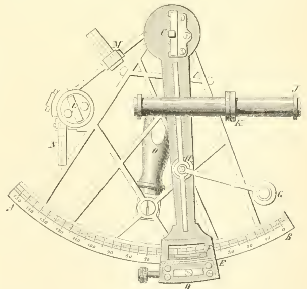
Nr. 5079. Der Spiegelsextant.
