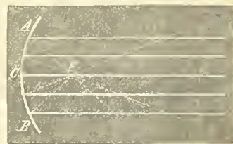
Nr. 5068. Zurückwerfung parallel auffallender Strahlen durch den Hohlspiegel.
