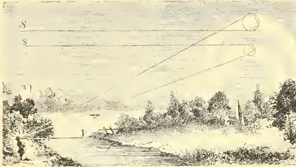
Nr. 4579. Zur Erklärung des Regenbogens.
