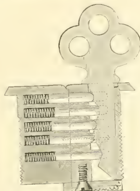
Nr. 4854. Vale's Sicherheitschloß. Längsdurchschnitt mit eingestecktem Schlüssel.
