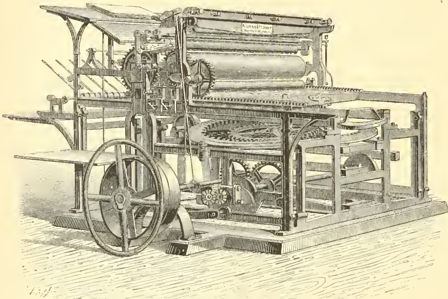
Kr 4886. Einfach Cylindermaschine mit Kreisbewegung. (System König & Bauer.)
